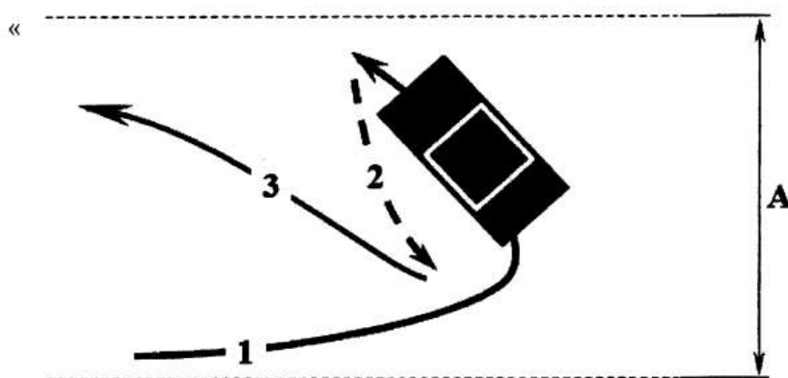
Рисунок 5. Схема маневра "Разворот транспортного средства в ограниченном пространстве (при ограниченной ширине проезжей части) с использованием движения задним ходом"
